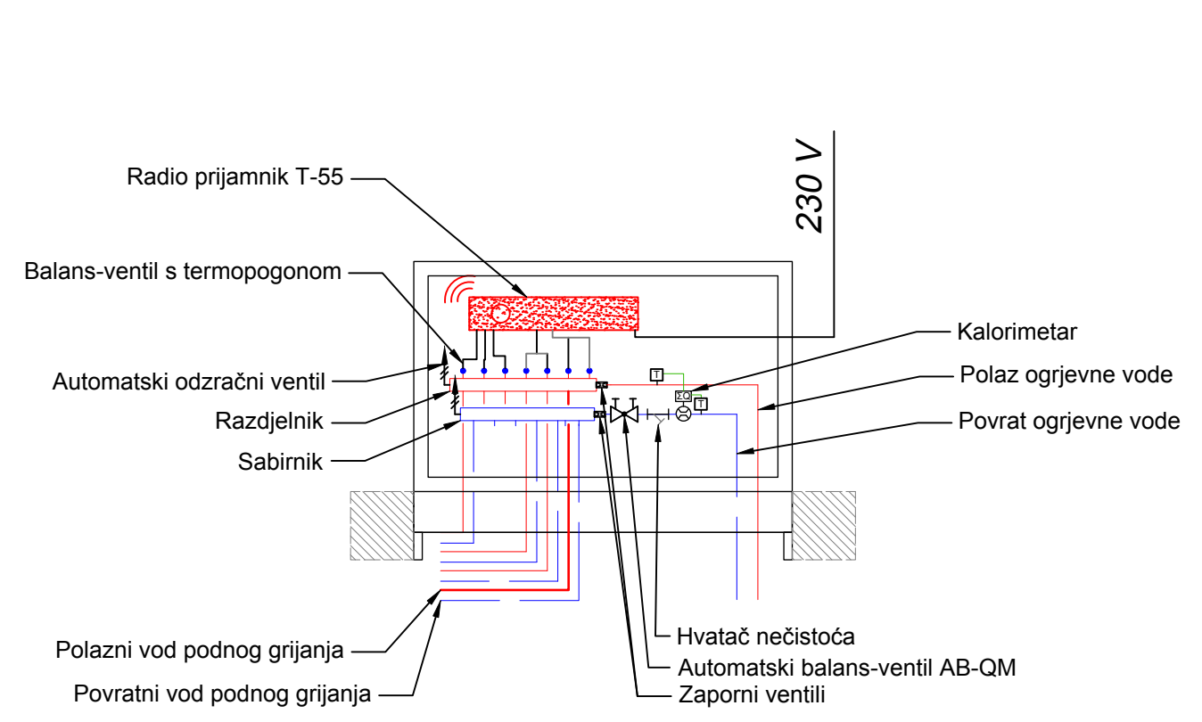
Primjer ormarića podnog grijanja s regulacijom
