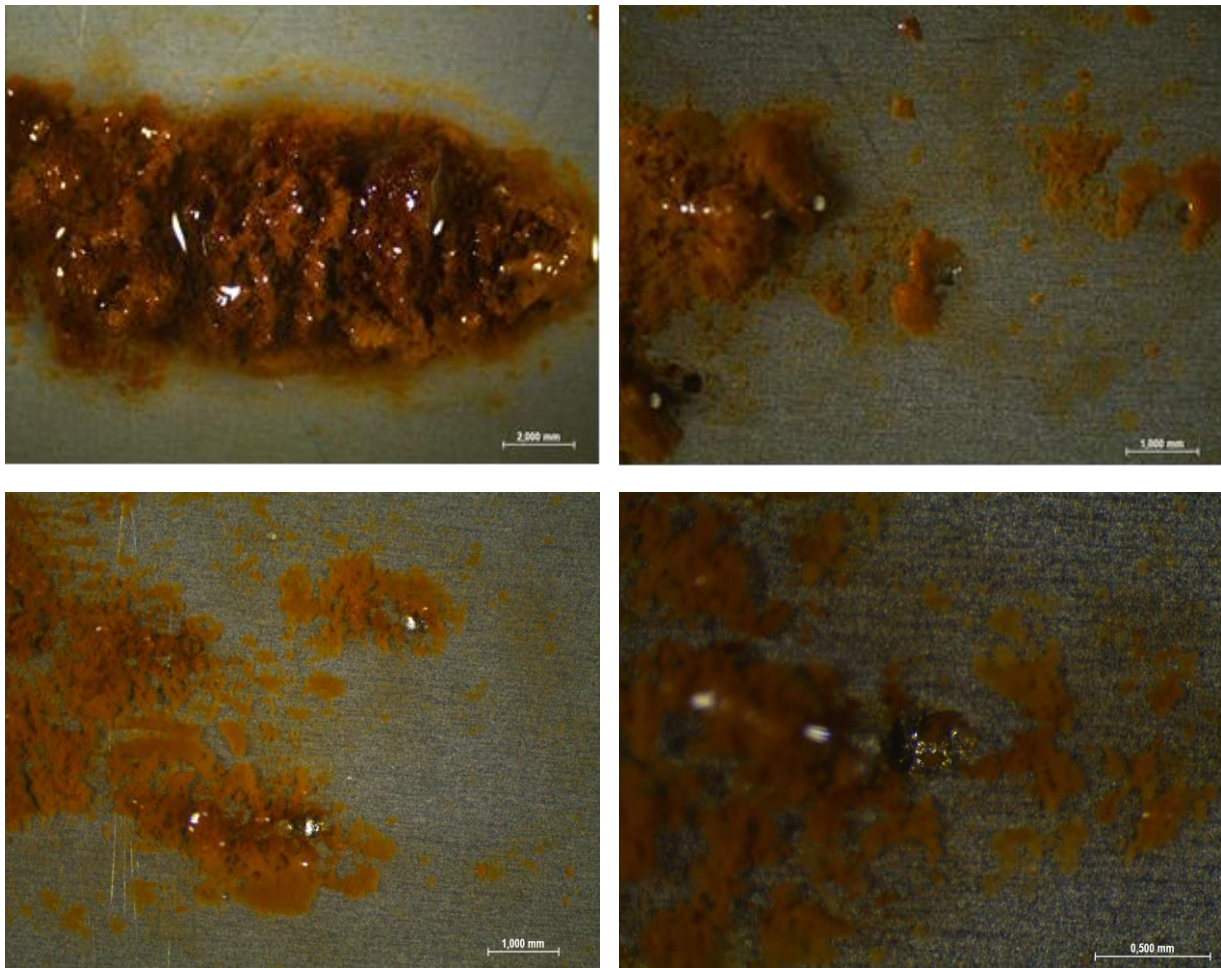
Slika 45. Stereomikroskopske snimke rupičaste korozije ispod korozijskih produkata na čeliku AISI 304L, nakon ispitivanja u 3,5 % otopini NaCl s dodatkom H_2O_2
