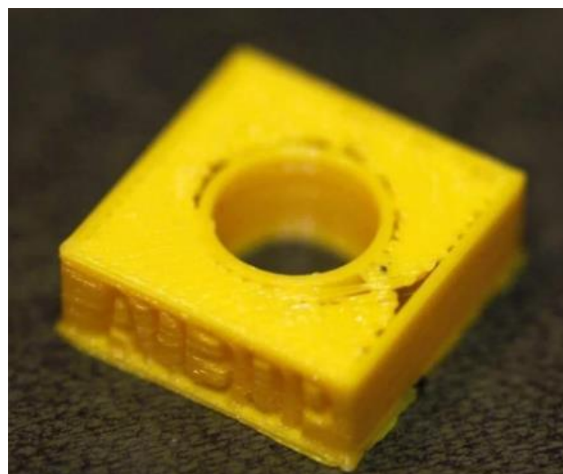
Slika 6. Narušena kvaliteta uslijed nepravilnog skupljanja materijala
