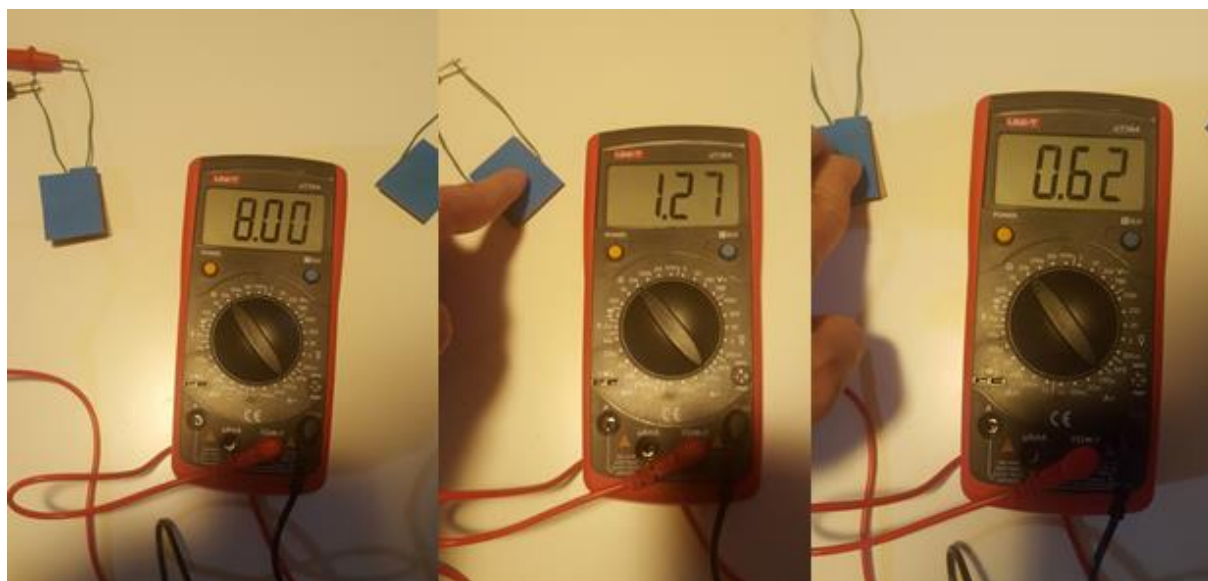
Slika 4. Otpor senzora
