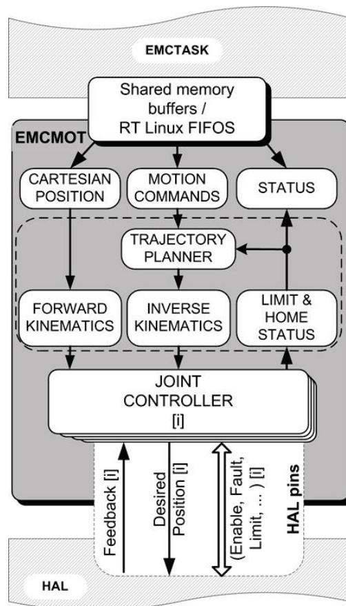
Slika 2. Struktura EMC MOT modula LinuxCNC-a [2]
