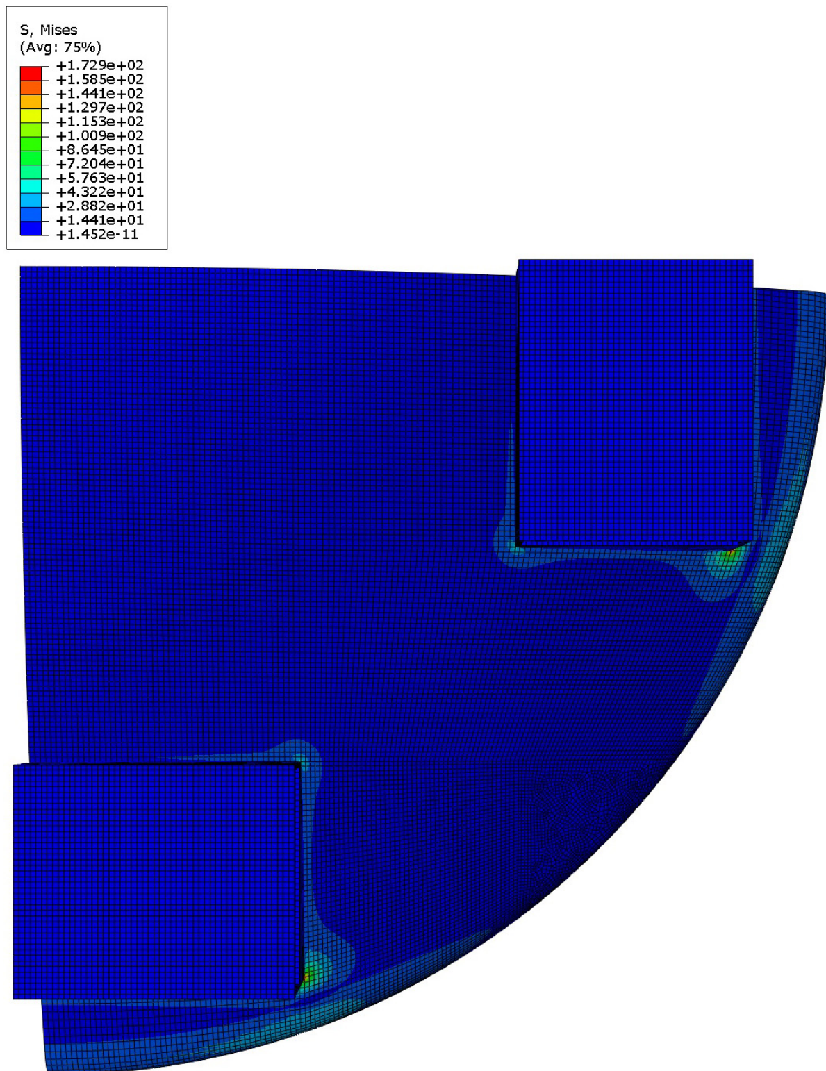
Slika 50. Naprežanje spremnika prema von Misesu
