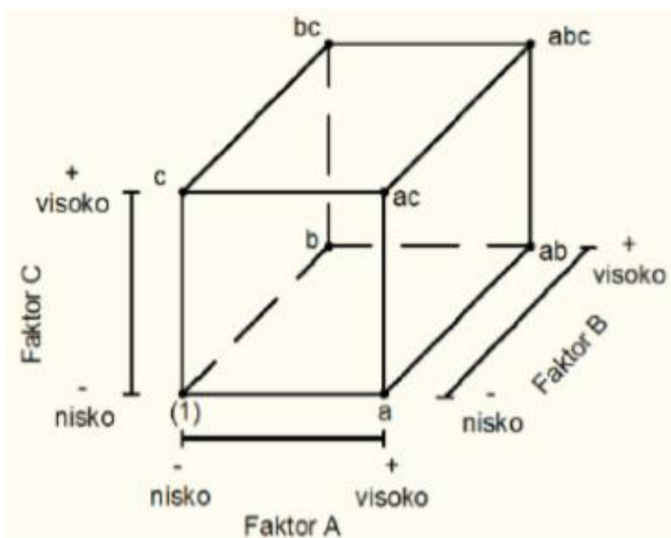
Slika 42. Grafički prikaz potpunog plana pokusa 2^3 [39]
