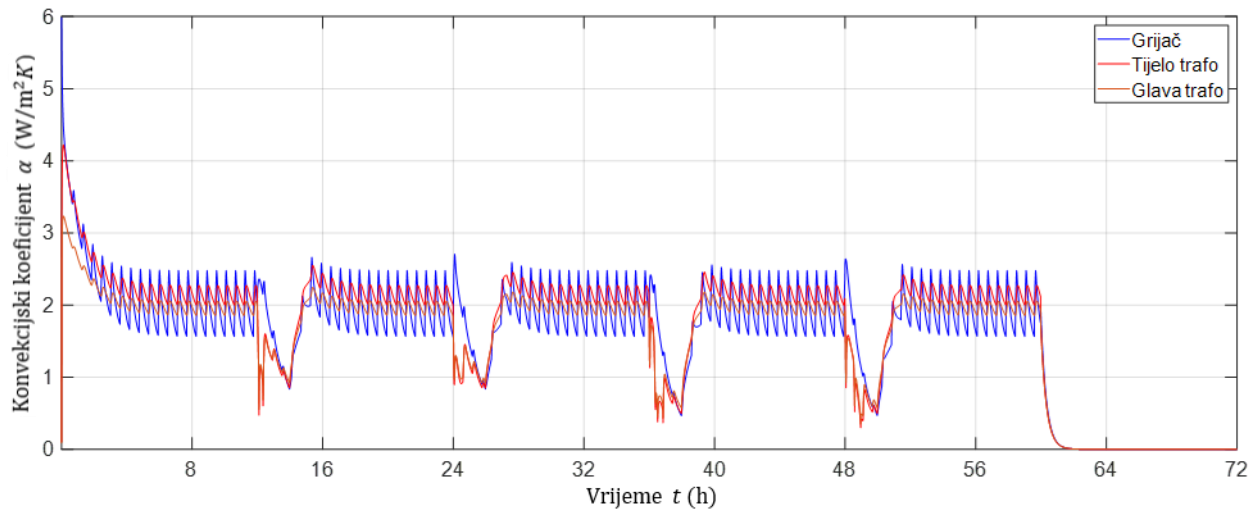
Slika 5.22. Koefficient prijelaza topline slobodne konvekcije s zraka na transformatore – slučaj 3
