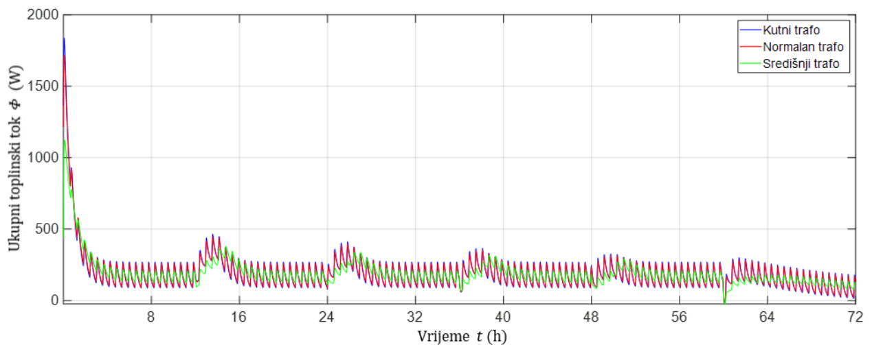
Slika 5.18. Ukupan dovedeni toplinski tok na izolaciju transformatora - slučaj 3
