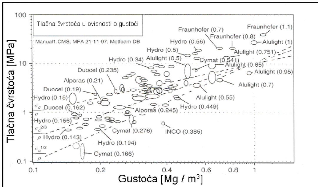
Slika 5.15. Prikaz vrijednosti tlačne čvrstoće u ovisnosti o gustoći za komercijalne metalne pjene. [7]
