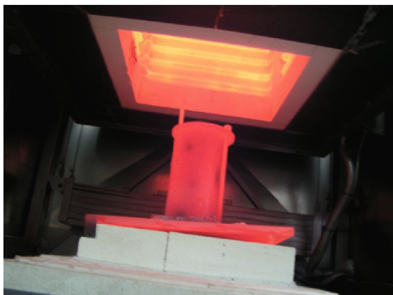
Slika 6.8. Izgled kalupa neposredno prije vađenja iz peći.
