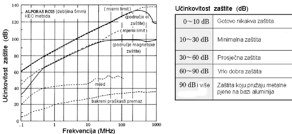
Slika 4.4. Dijagramski prikaz učinkovitosti zaštite (os ordinata) o frekvencijskom rasponu (os apscisa). [5]
