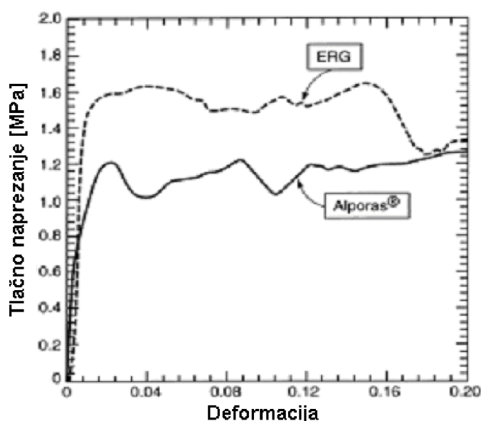
Slika 5.13. Dijagram naprezanje-deformacija otvorenih (ERG) i zatvorenih (Alporas) metalnih pjena. [7]
