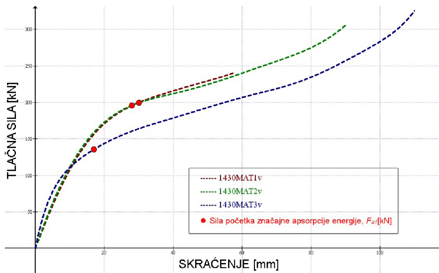
Slika 6.25. Dijagram TLAČNA SILA – SKRAĆENJE s ucrtanim točkama početka i završetka apsorpcije energije za uzorke 1430MAT i brzinu ispitivanja v_2 = 60\text{mm/min} .
