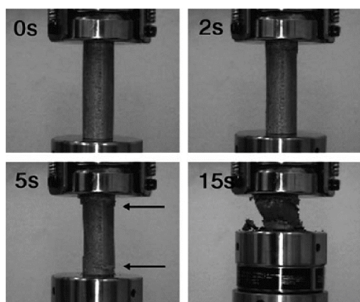
Slika 5.4. Prikaz tlačnog loma prilikom tlačenja nakon 2, 5 i 15s uzorka visine 60mm. [6]
