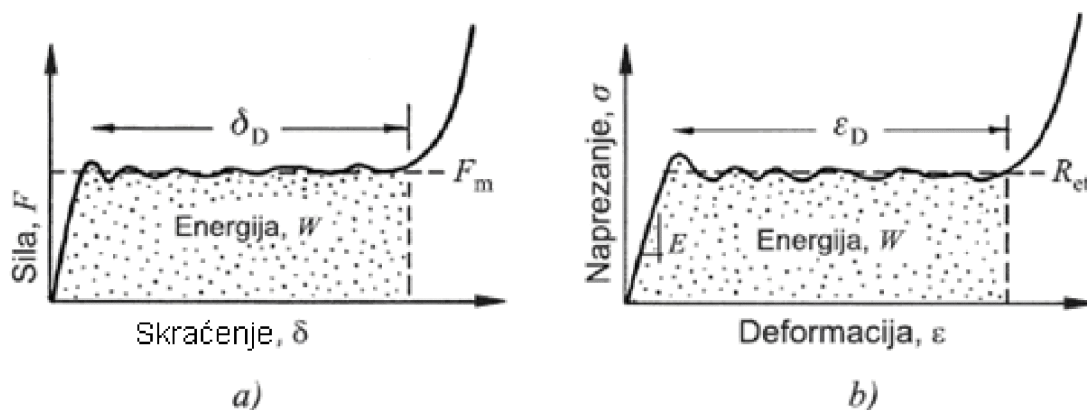
Slika 6.20. Apsorbirana energija prikazana kao površina ispod krivulje: c) u dijagramu SILA – SKRAĆENJE d) u dijagramu NAPREZANJE - DEFORMACIJA
