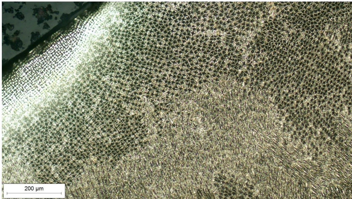
Slika 31. Tjeme metala zavara snimljeno pri povećanju 100×
