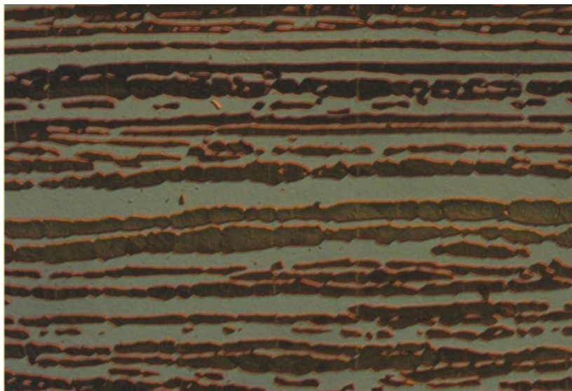
Slika 8. Mikrostruktura dupleks čelika [12]
