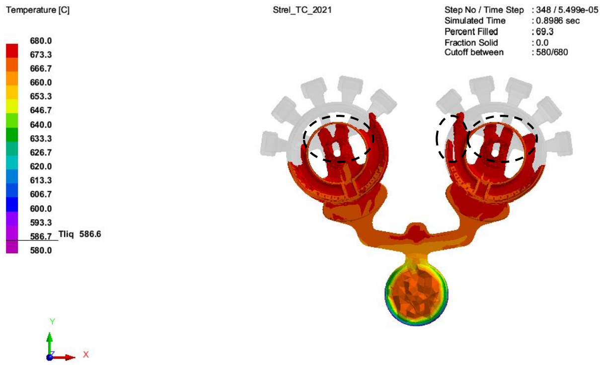
Slika 36. Prikaz punjenja kalupa pri 61,9% popunjenosti 2.
