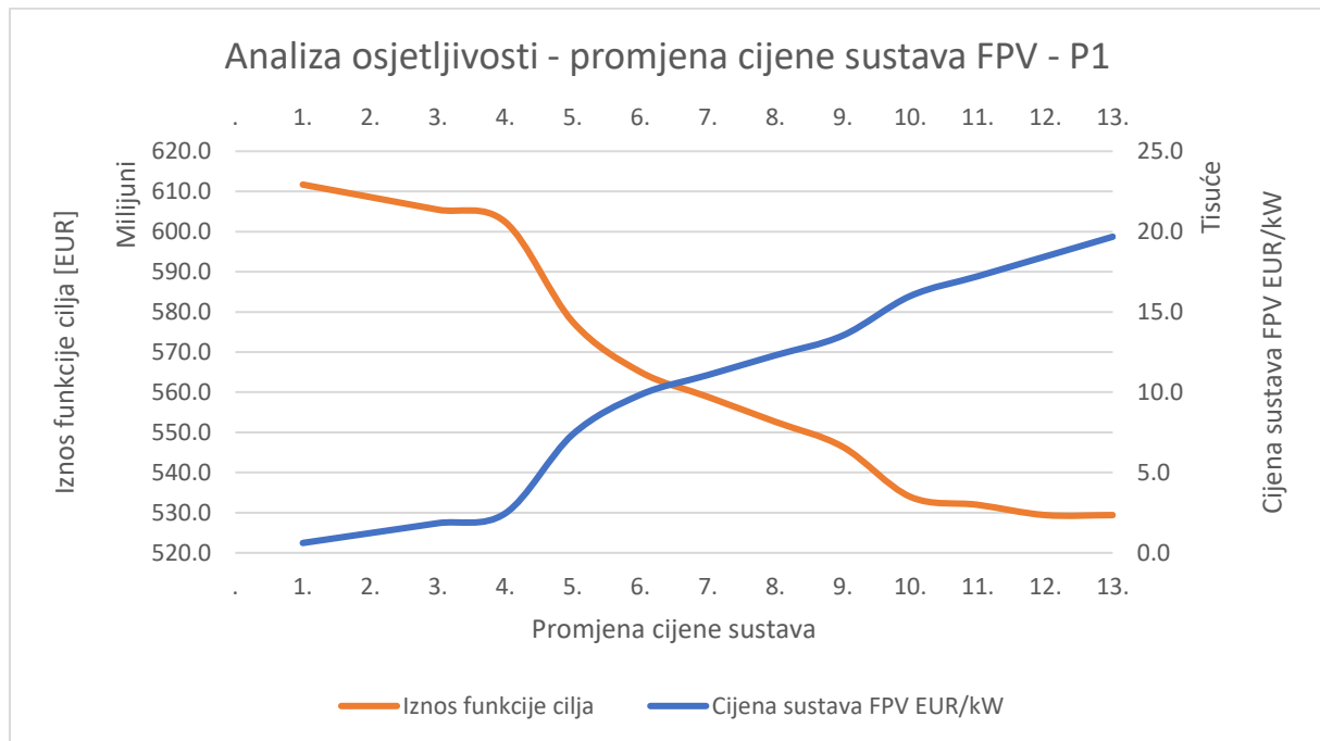
Graf 22. Analiza osjetljivosti - promjena cijene sustava FPV - P1
