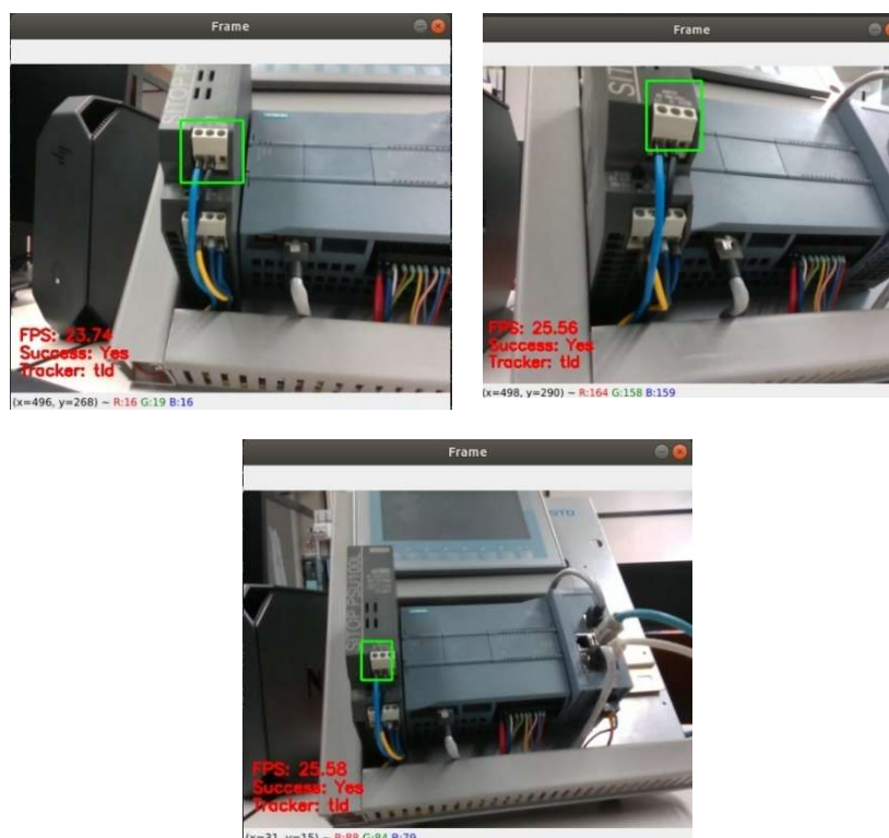
Slika 21. Praćenje rednih stezaljki PLC-a pomoću TLD algoritma praćenja
