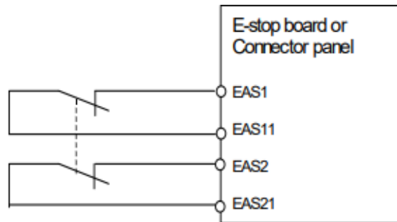
Slika 14: E-Stop priključnice[6]
