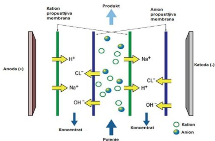
Slika 2.3 Shematski prikaz ED procesa [7]
