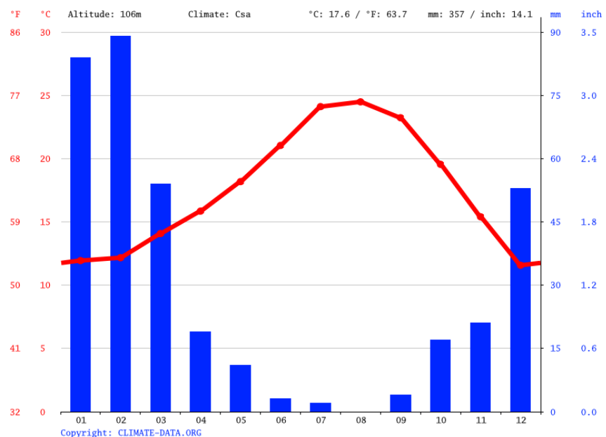
Slika 4. Temperatura i padaline po mjesecima Los Angeles
