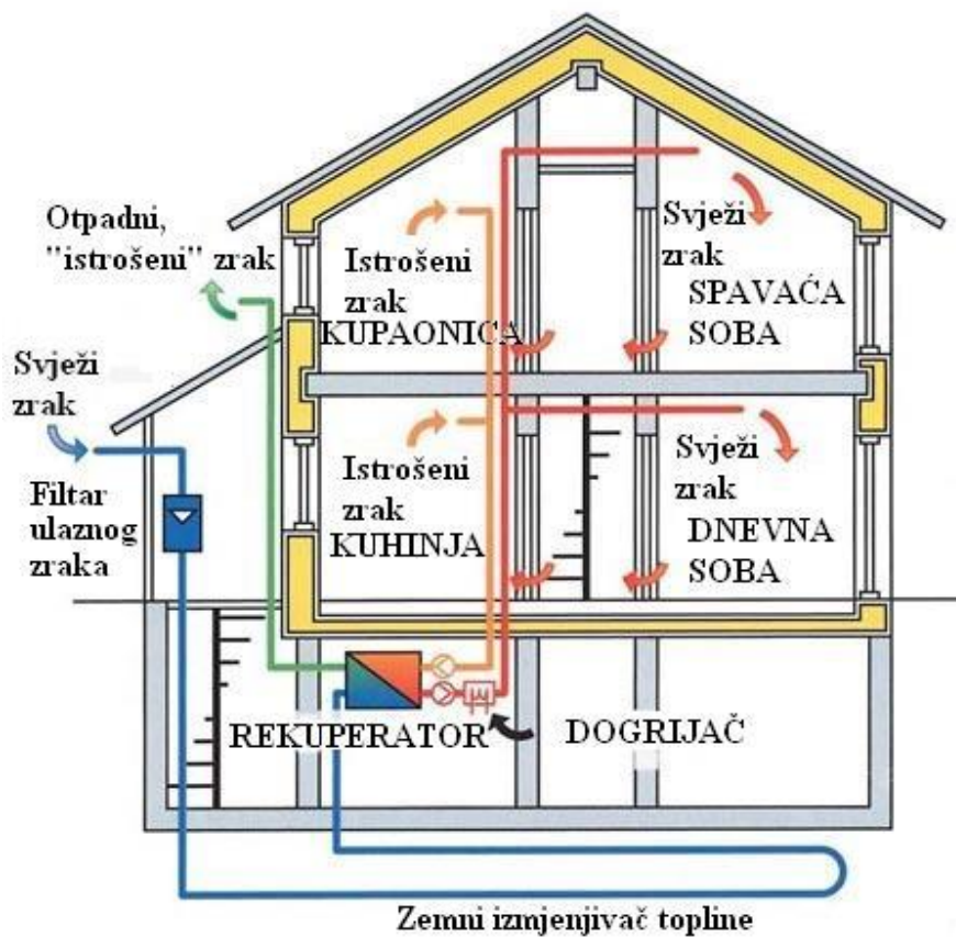
Slika 17. Ventilacija pasivne kuće
