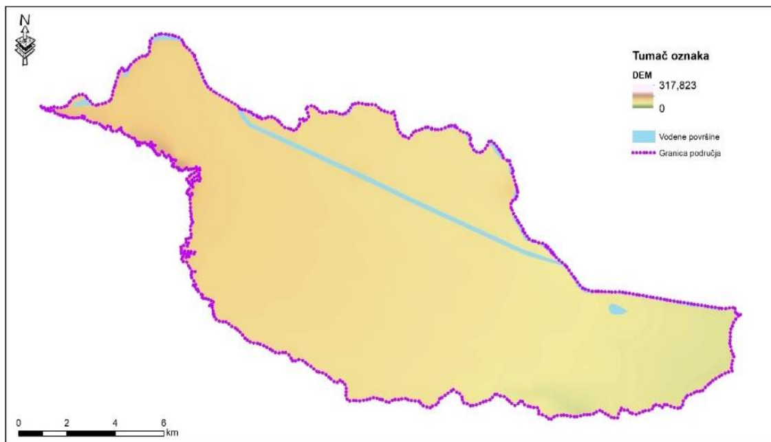
Slika 4.1. DMR raster
