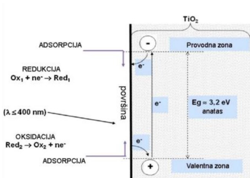
Slika 2. Proces fotokatalitičke reakcije [7]
