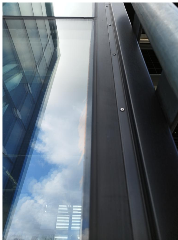
Slika 28 Primjer korodiranog low-E premaza
