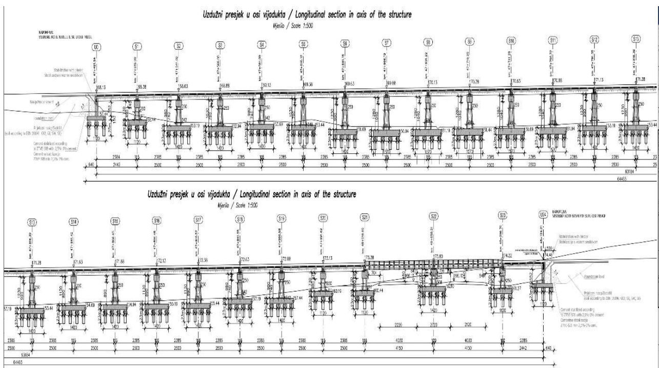
Slika 15: Uzdužni presjek vijadukta Carevdar (Izvor: [3])
