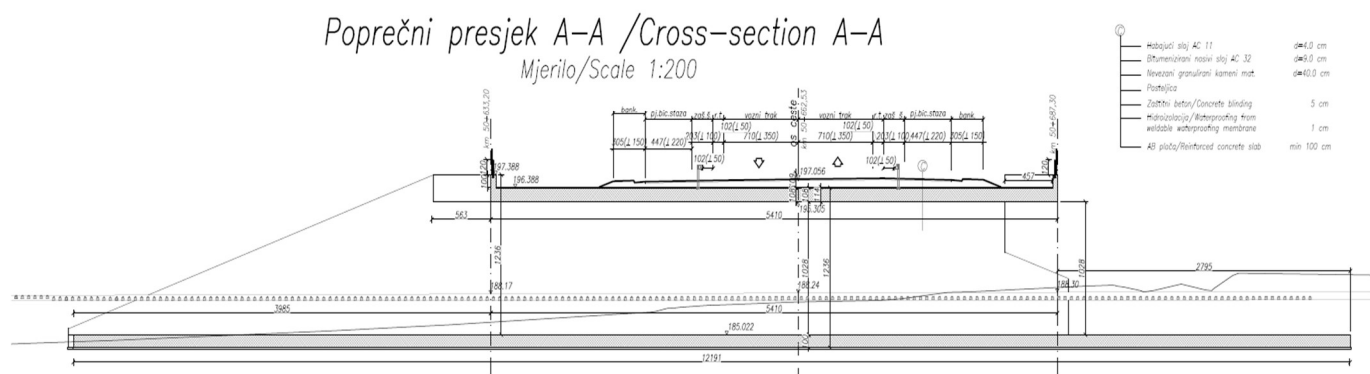
Slika 17: Poprečni presjek nadvožnjaka Lepavina 1 (Izvor: [4])
