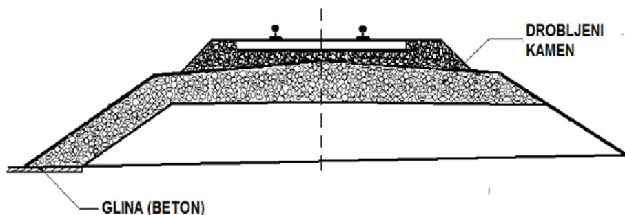
Slika 52: Gotova prokapnica (Izvor: [8])
