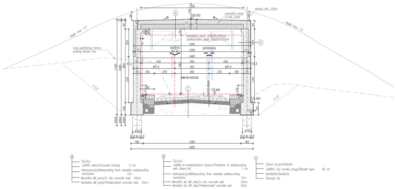
Slika 28: Poprečni presjek galerije Velika Mučna (Izvor: [6])
