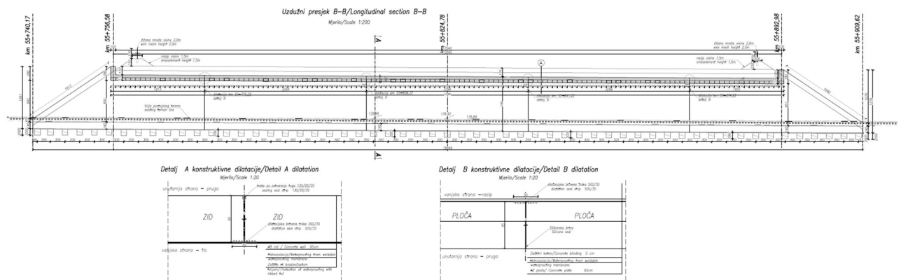
Slika 29: Uzdužni presjek galerije Velika Mučna (Izvor: [6])
