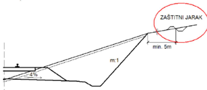
Slika 66: Odvodni i zaštitini jarak (Izvor: [8])
