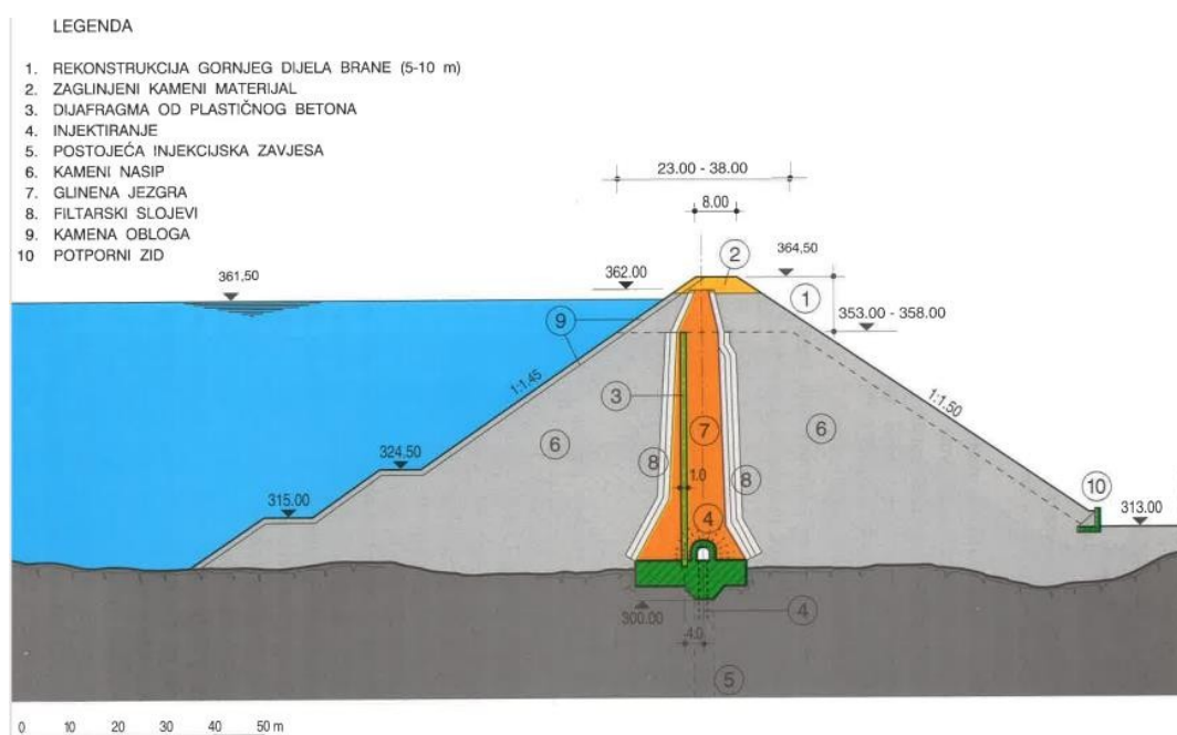
Slika 15: Poprečni presjek rekonstrukcije brane s dijafragmom od plastičnog betona (Izvor: [10])
