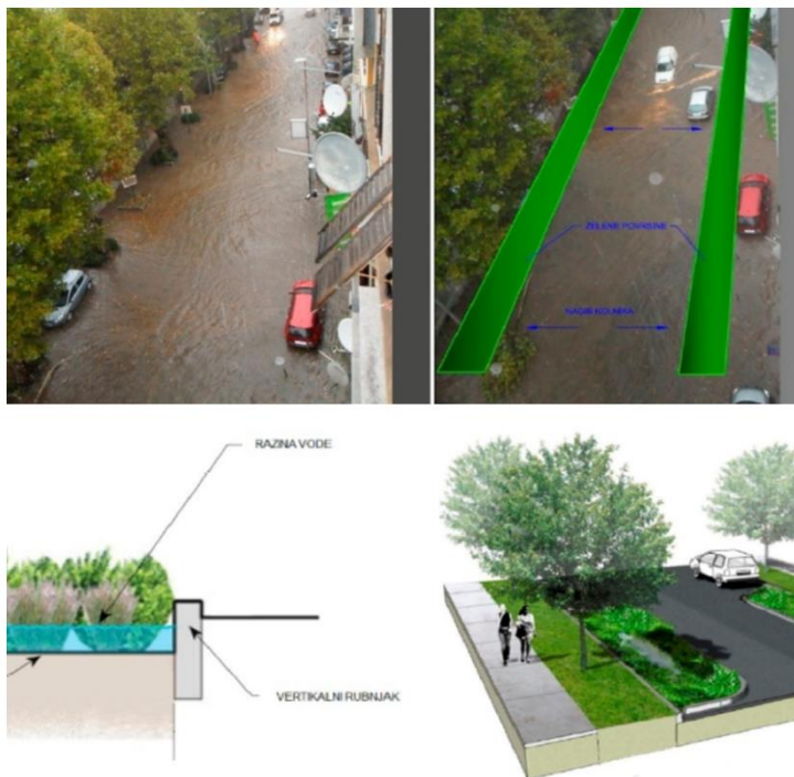
Slika 17.: Prikaz primjene rješenja zelene infrastrukture u Gradu Rijeci (Izvor: [6])
