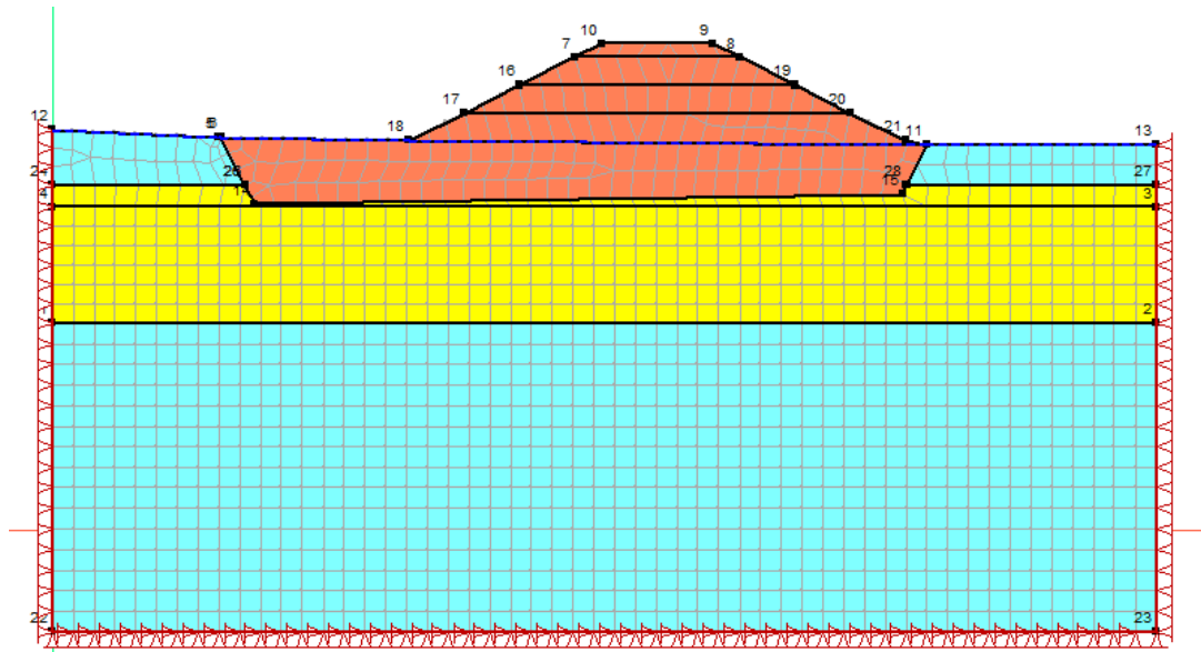
Slika 72. Zadavanje materijala-geotehnička sredina pijesak (SC) plići položaj
