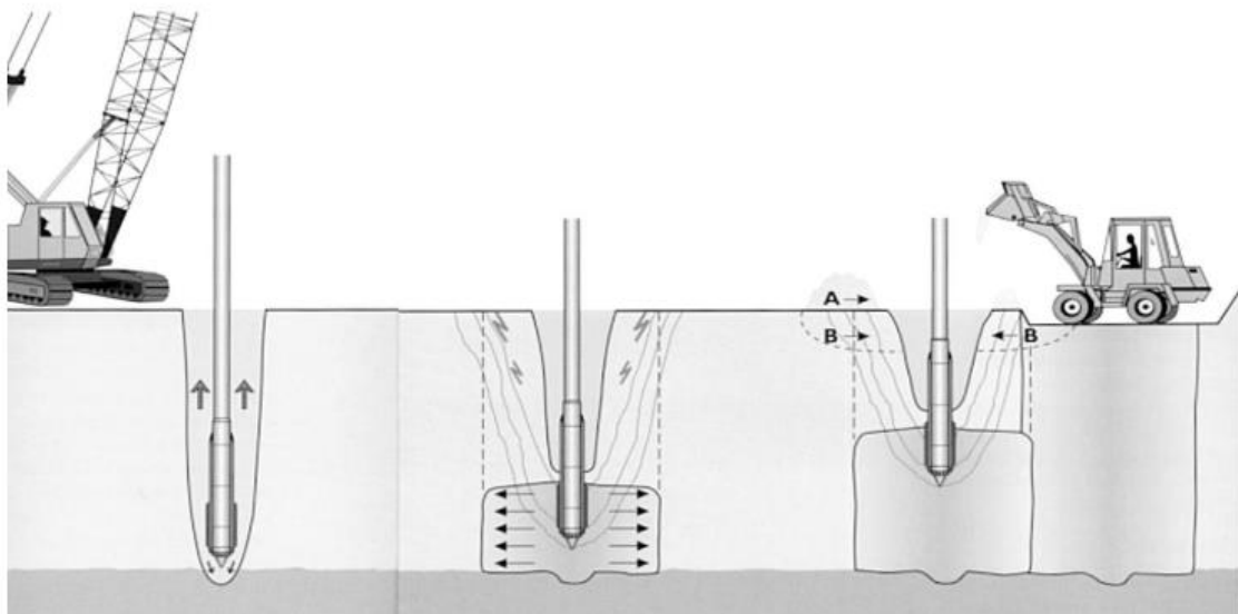
Slika 12.:Princip izvođenja vibracijskog zbijanja (Izvor: [9])
