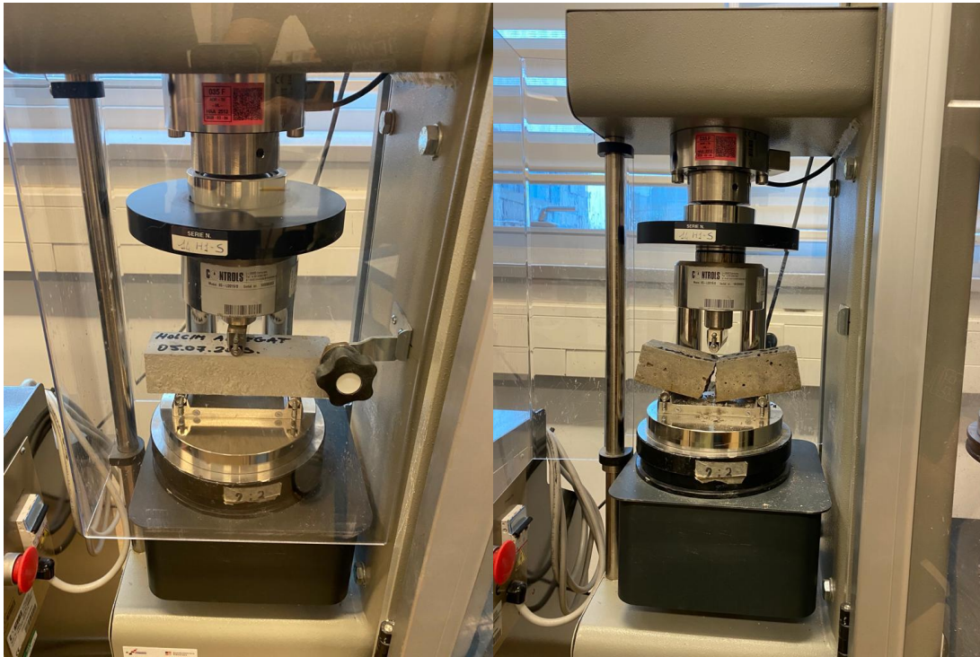
Slika 25. Ispitivanje vlačne čvrstoće savijanjem
