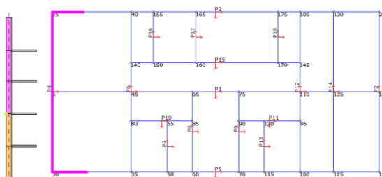
Slika 87. Geometrija pretpostavljenog bloka mehanizma otkazivanja B2 (gore), prikaz položaja zgloba (dolje lijevo), položaj zida u konstrukciji (dolje desno)
