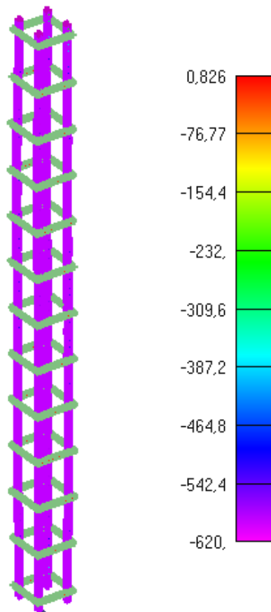
Slika 6.265: Prikaz naprezanja glavne uzdužne armature za djelovanje požara od 120min KRAJ ZAGRIJAVANJA I POČETAK HLAĐENJA (NAKON OVOG TRENUTKA STUP SE VRLO BRZO SRUŠIO)
