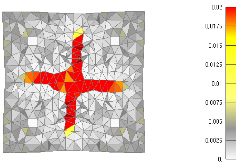
Slika 6.47: Prikaz pukotina za poprečni presjek stupa nakon 90 minuta požara (gore-sa sponama, dolje-bez spona)
