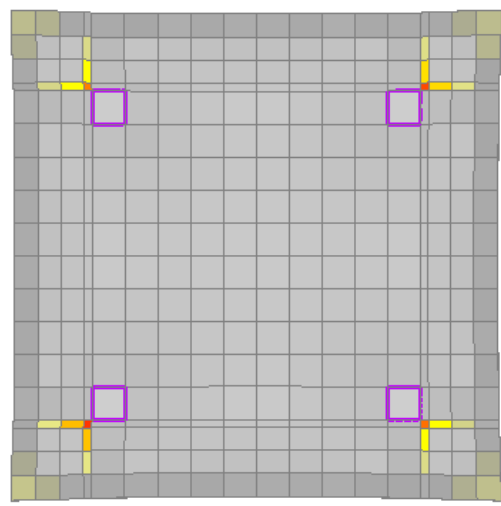
Slika 6.107: Prikaz pukotina za poprečni presjek stupa nakon 30 minuta požara (gore-sa sponama, dolje-bez spona)
