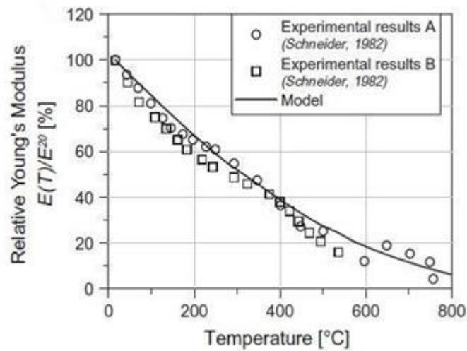
Slika 2.3: Prikaz Young-ovog modula elastičnosti u ovisnosti o temperaturi
