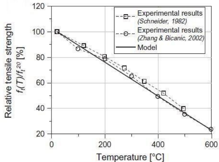
Slika 2.2. Prikaz vlačne čvrstoće u ovisnosti o temperaturi
