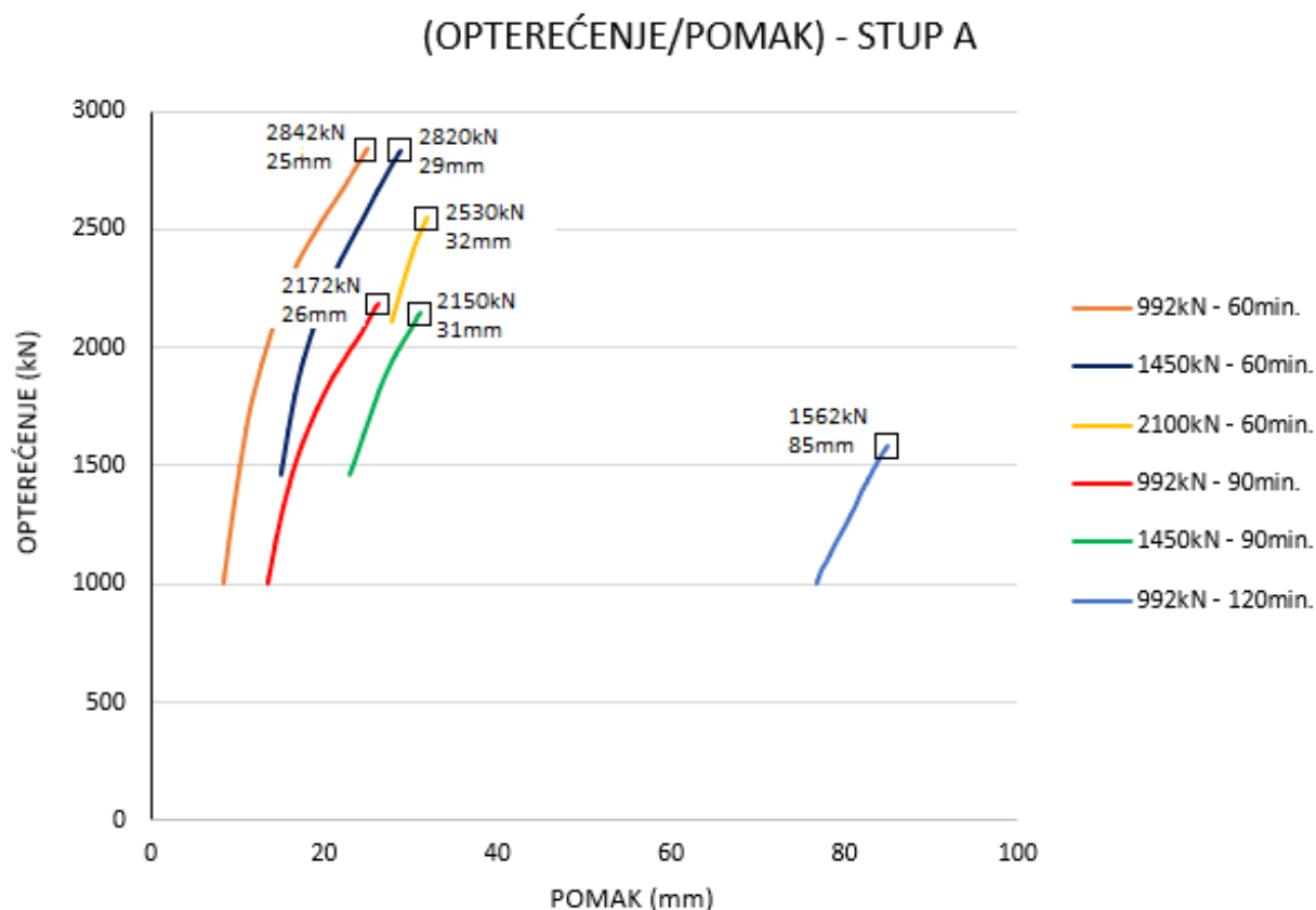
Slika 6.283: Prikaz dijagrama (opterećenje-pomak) i sile sloma stupova za kombinacije iz parametarske studije
