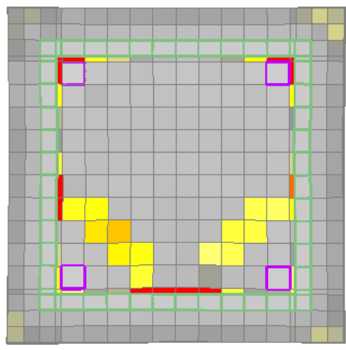
Slika 6.108: Prikaz pukotina za poprečni presjek stupa nakon 60 minuta požara (sa sponama) (KRAJ ZAGRIJAVANJA I POČETAK HLAĐENJA)
