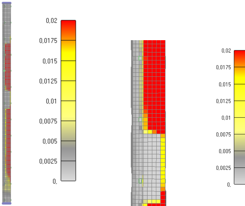
Slika 6.179: Prikaz pukotina za jednu četvrtinu stupa nakon 90 minuta (lijevo-cijeli stup, desno-detalj stupa) -KRAJ GRIJANJA I POČETAK HLAĐENJA
