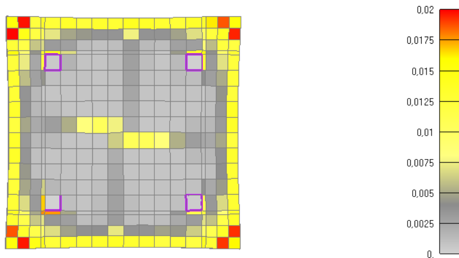
Slika 6.84: Prikaz pukotina za poprečni presjek stupa nakon 175 minuta požara (gore-sa sponama, dolje-bez spona)-KRAJ LINEARNOG I POČETAK KONSTANTNOG HLAĐENJA
