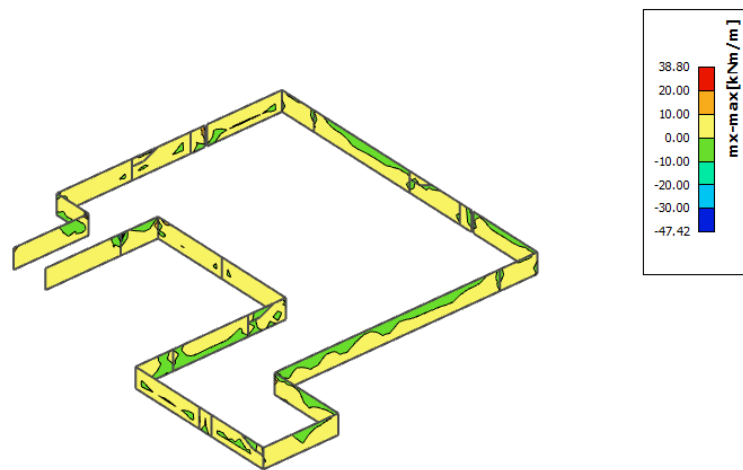
Slika 15.3. M_x
