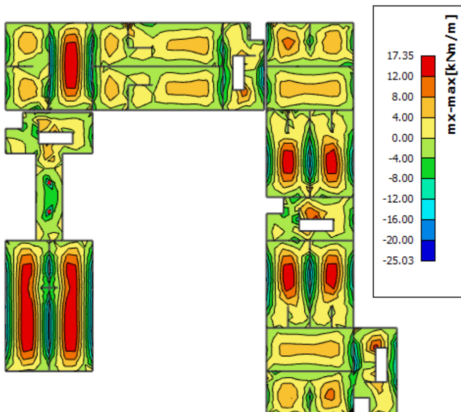
Slika 11.18. M_x
