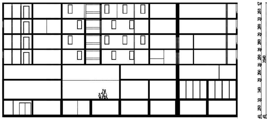
Slika 1.3. Presjek A-A
