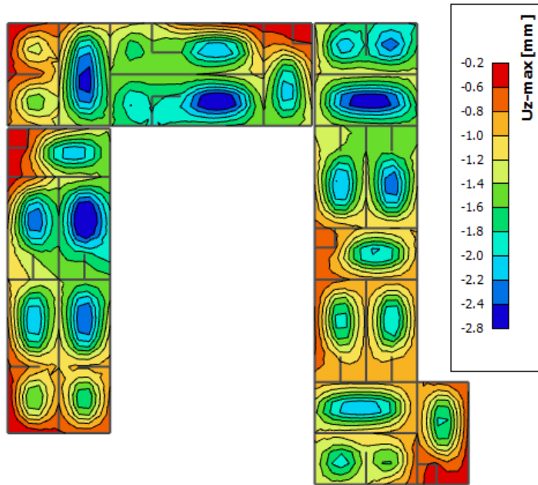
Slika 11.7. Prikaz progiba
