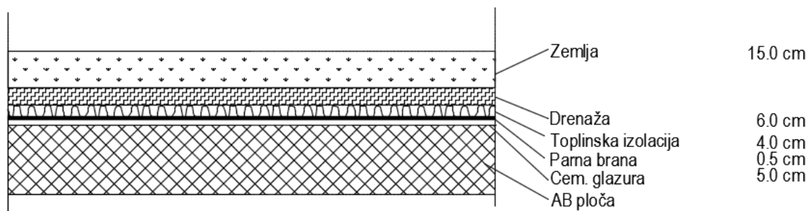
Slika 8.4. Slojevi poda
