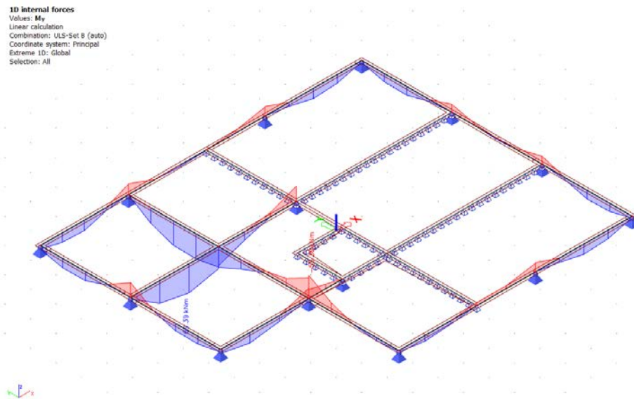
Slika 52 Dijagrami momenata savijanja M_y na gredama
