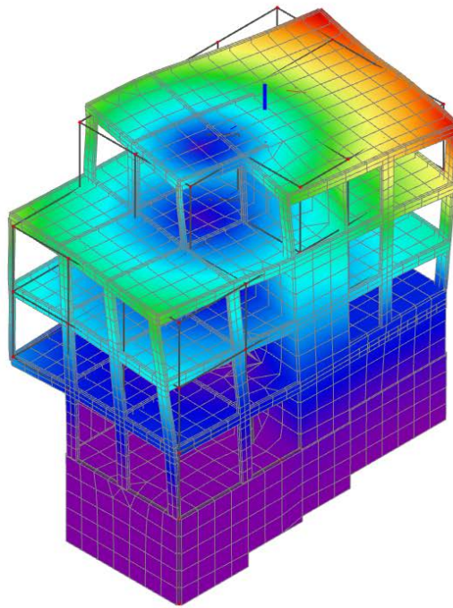
Slika 45 Torzija oko globalne osi Z (2)
