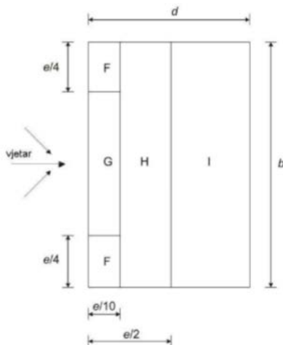
Slika 21 Raspored polja za ravne krovove
