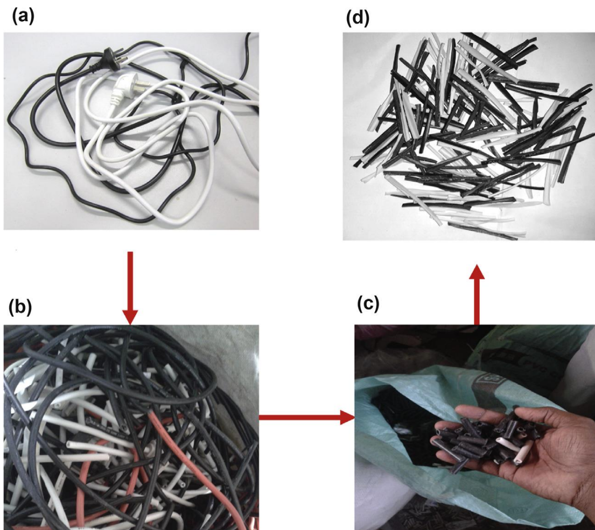
Slika 19 Postupak proizvodnje PVC vlakana od e-otpada. (a) Odbačeni električni PVC kabele. (b) PVC vlakna. (c) Vanjska ovojnica PVC kabela nakon uporabe metala. (d) Vanjska ovojnica PVC-a izrezana na male dužine. [2]
