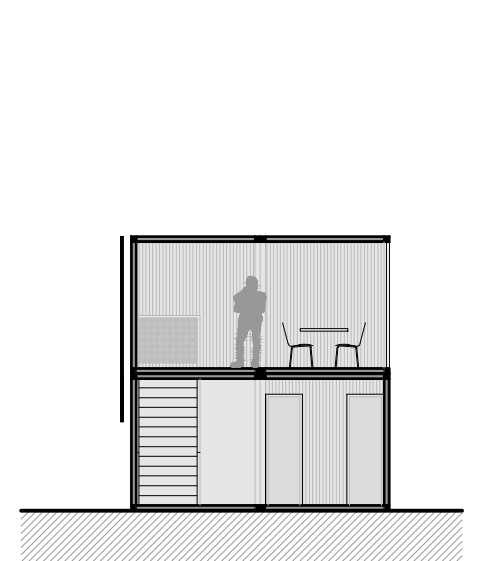
presjek
