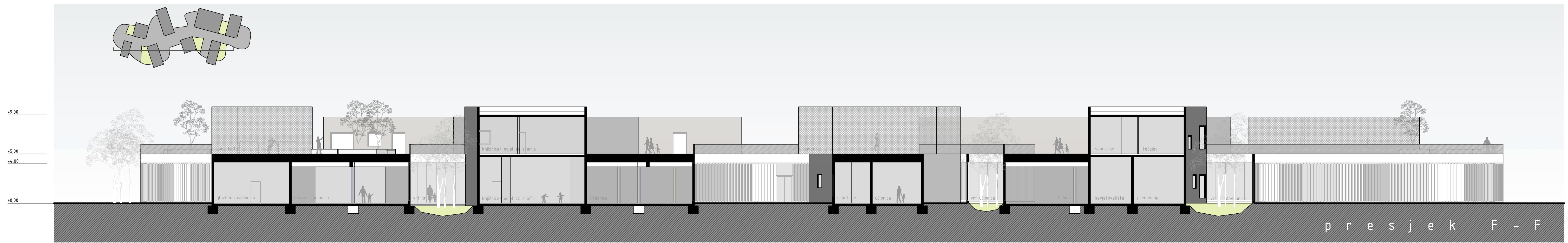
presjek E - E
