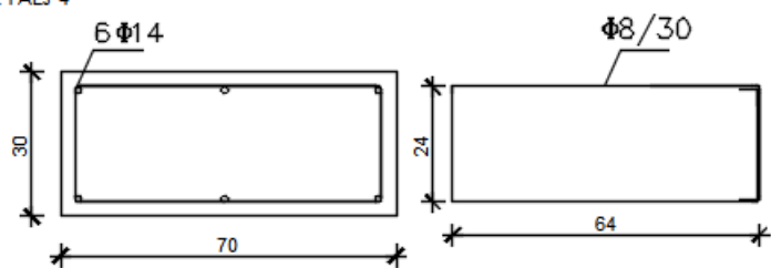
DETALJ 4
