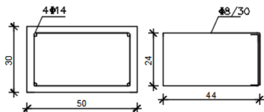
DETALJ 5
