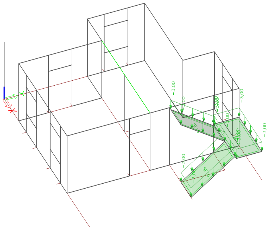
Slika 4.5 Dodatno stalno djelovanje G_1 ( \text{kN/m}^2 )
