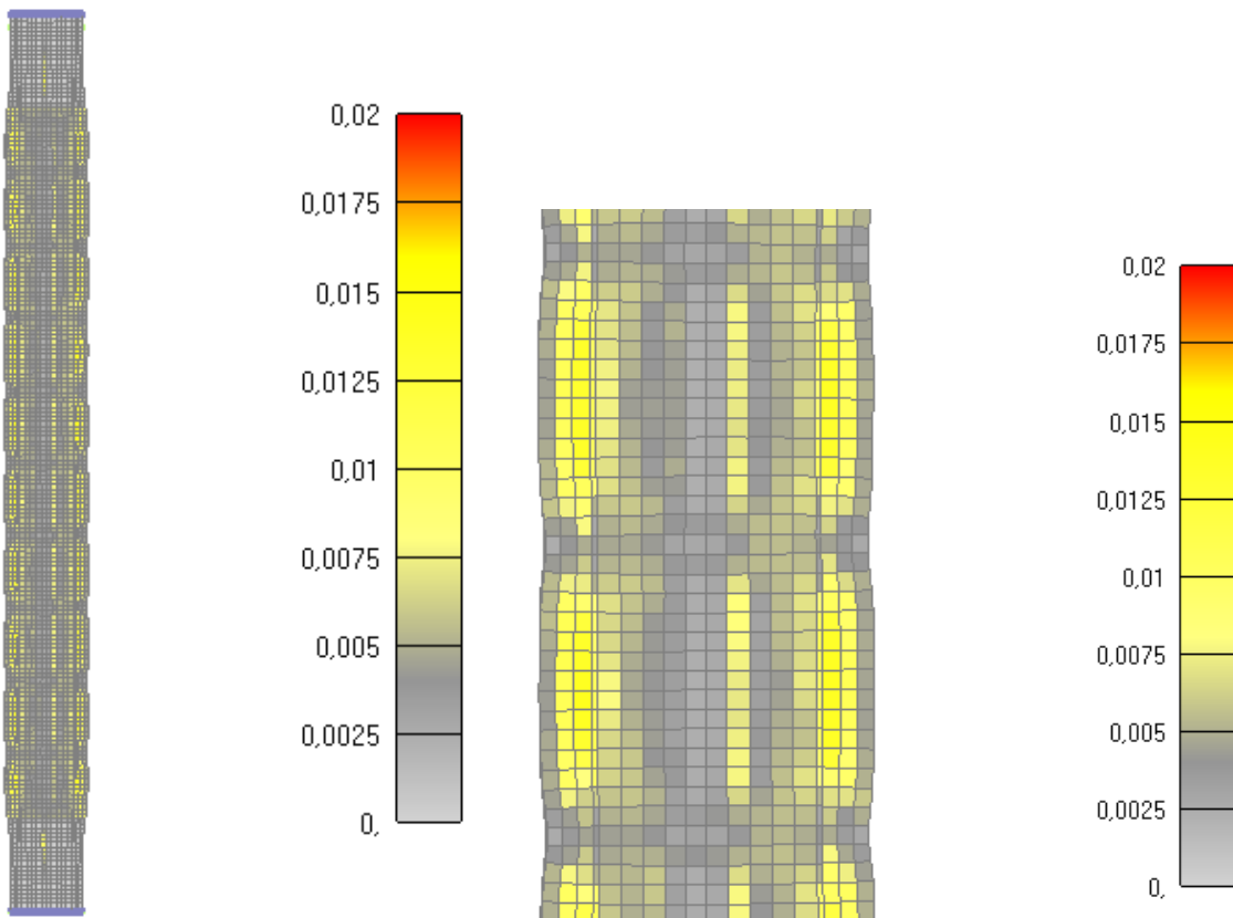
Slika 6.239: Prikaz pukotina za cijeli stup nakon 120 minuta ( lijevo-cijeli stup, desno-detalj stupa ) -KRAJ GRIJANJA I POČETAK HLADENJA
