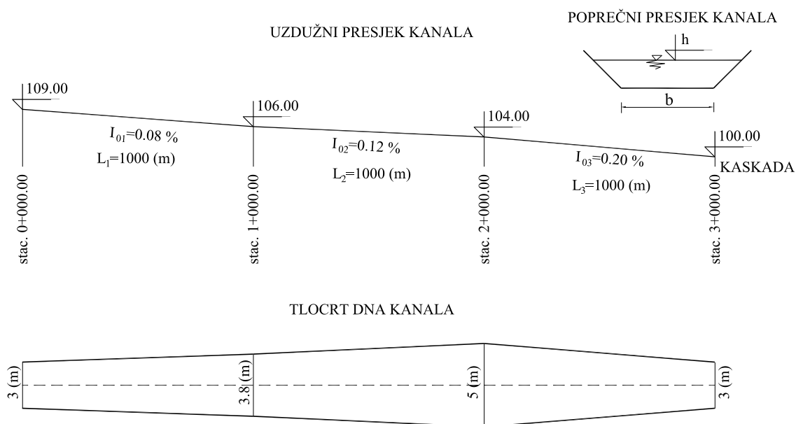
Slika 1. Geometrija kanala
