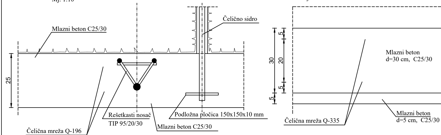
RAZVIJENI PRESJEK REŠETKASTIH NOSAČA I SIDARA
