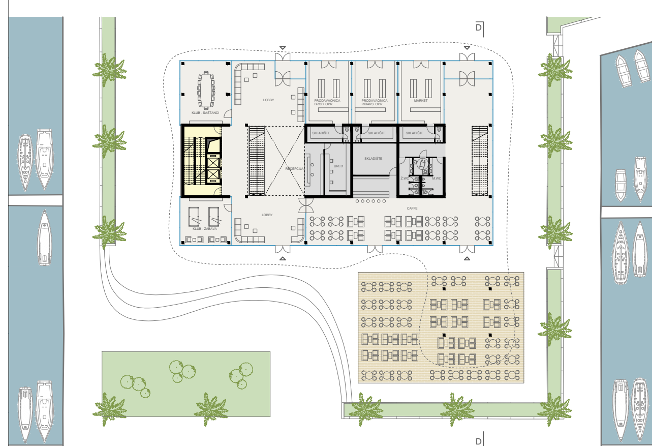
TLOCRT PRIZEMLJA
