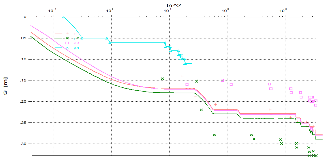
Slika 4.32 – S - t/r^2 (log) za piezometre na radijusu R=11,2 m
