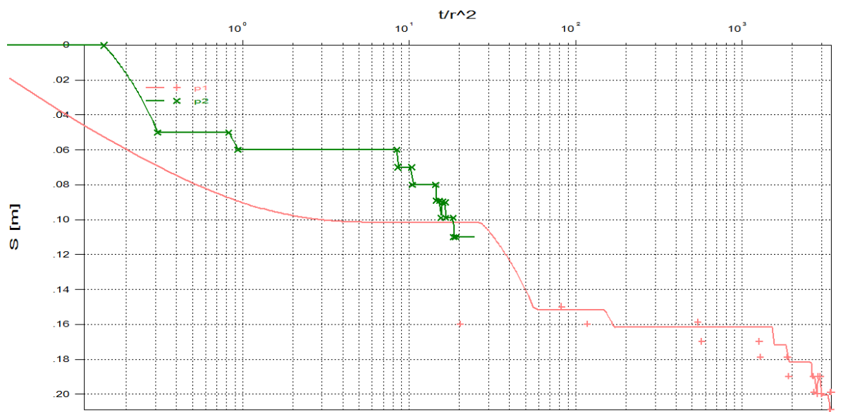
Slika 4.22 – S - t/r^2 (log) za piezometar R=11,2 m i Z=15,5 m
