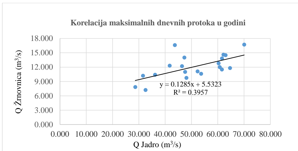
Slika 9.1.2. Korelacija maksimalnih dnevnih protoka Jadra i Žrnovnice za razdoblje 1995.-2014.
