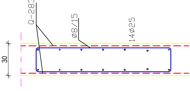
Detalj B
