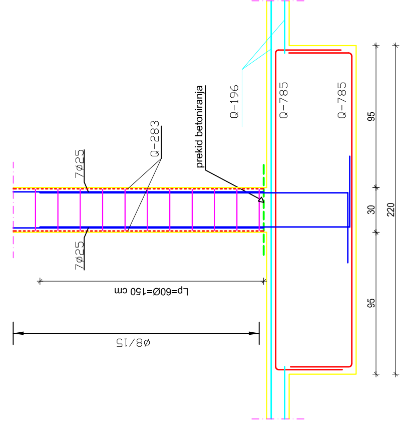
PRESJEK B-B
