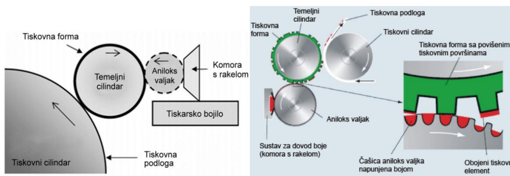
Slika 4.20 Princip rada fleksotiska[13]
