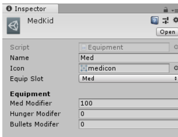
Slika 23. Predložak
