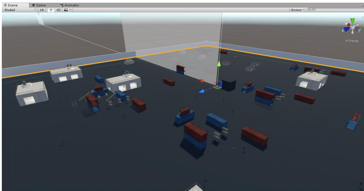
Slika 4. Scene View
