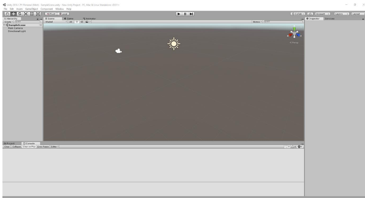
Slika 2. Sučelje Unity-a
