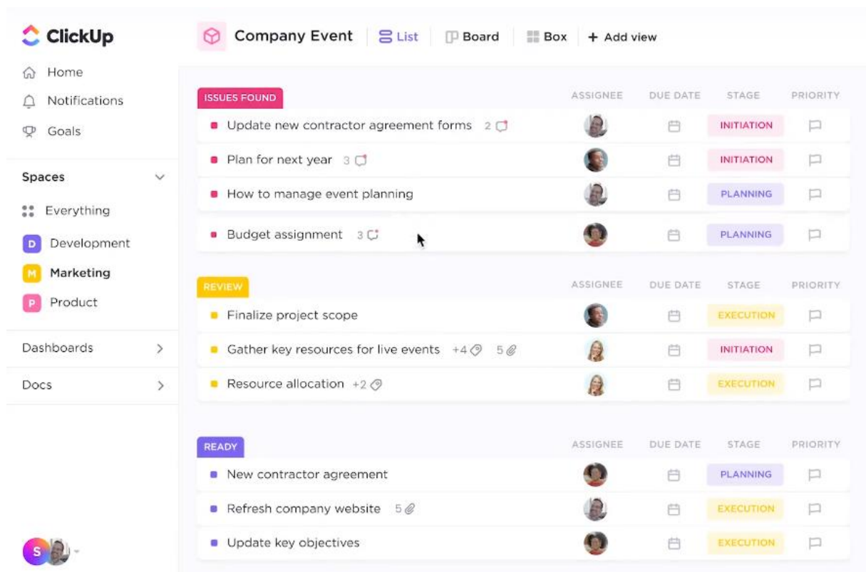
Slika 1: ClickUp UI
