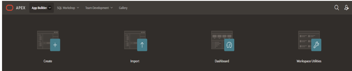
Slika 22: Kreiranje aplikacije
