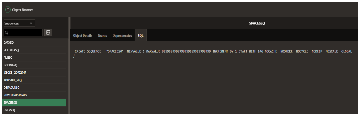
Slika 14: Sekvenca
