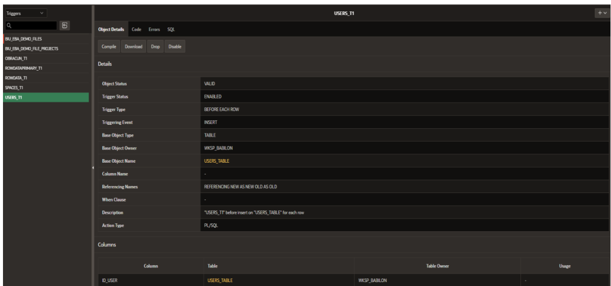
Slika 15: Trigger
