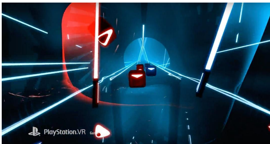
Slika 8 Beat Saber
