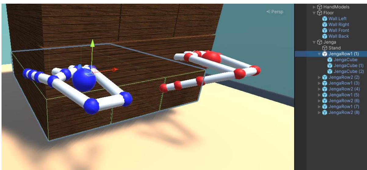
Slika 20 JengaRow prefarbi
