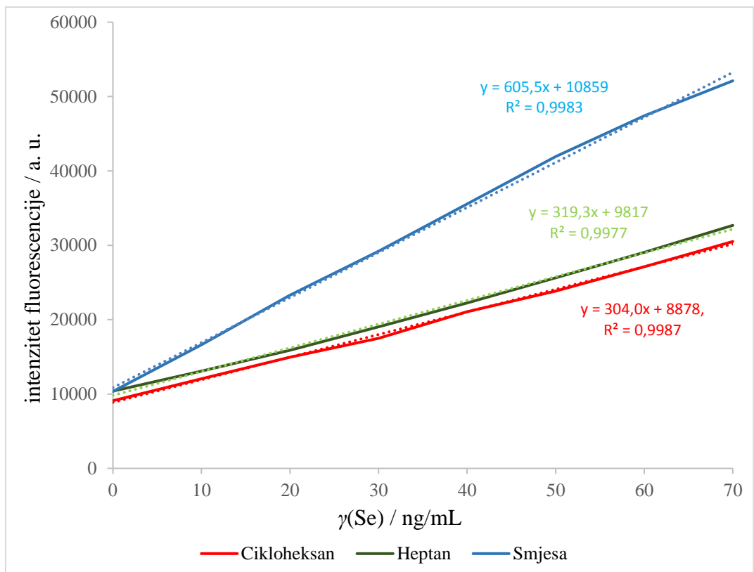
Slika 24. Grafički prikaz ovisnosti intenziteta fluorescencije o koncentraciji selenija u kompleksu Se-DAN u cikloheksanu, heptanu i smjesi heptana i 3%- n -butil-acetata kao otapalu
