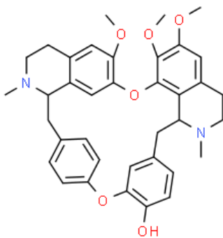
Slika 22. Struktura berbamina [67].
