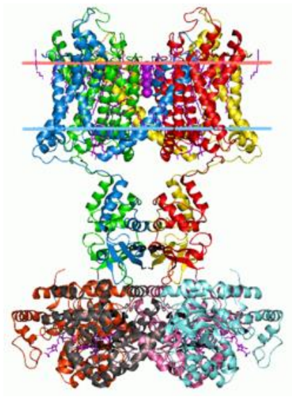
Slika 3. Tip kalijevog kanala. Na slici se mogu vidjeti sekundarna, tercijska i kvaterna struktura proteina. 17
