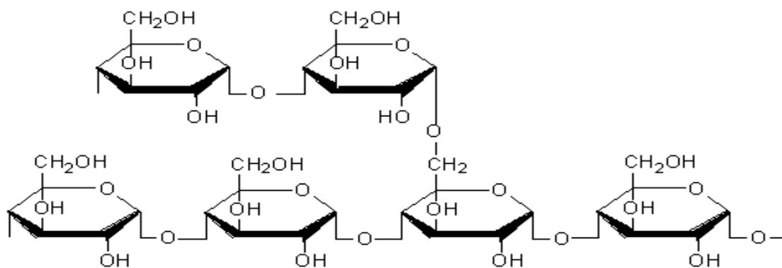
Slika 4. Struktura amilopektina
