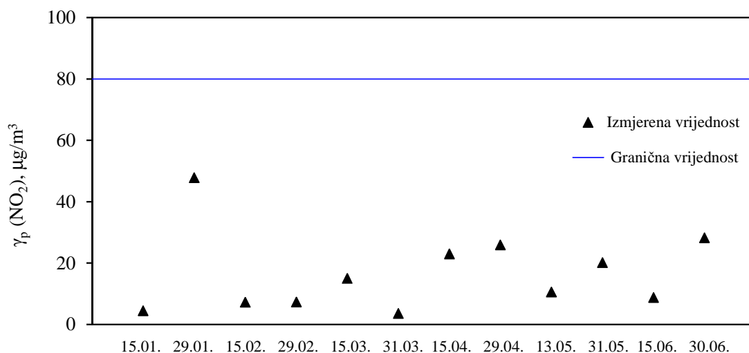
Slika 4.5. Usporedba graničnih i tolerantnih vrijednosti emisija s izmjerenim vrijednostima emisija koncentracija NO 2 na mjernoj lokaciji Zavoda za javno zdravstvo u Splitu za šestomjesečni mjerni period.
